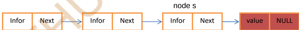
Hình 3.3. Thêm node vào cuối danh sách liên kết đơn
